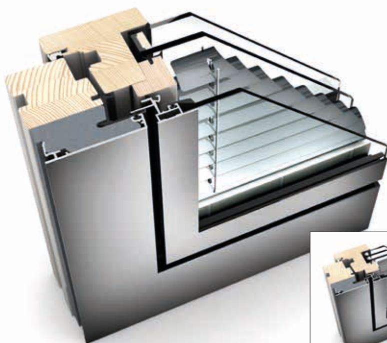
Triplo vetro opzionale + lastra singola
