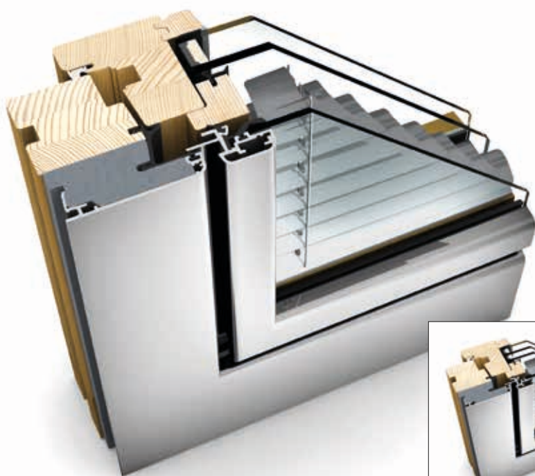
Tripla vetro opzionale + lastra singola
